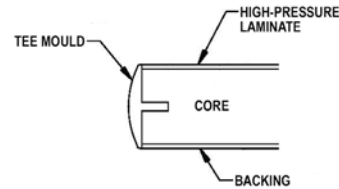
Edge Detail
