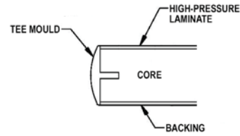
Edge Detail
