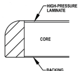
Abridge Drop Edge Band
